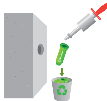
PASO 7: Arroja ambas partes del RivePipe dentro del cubo para su posterior re-utilización
