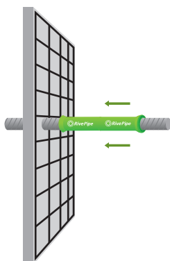
PASO 2: RivePipe protege las varillas o espadines del hormigón cuando se insertan entre los paneles
