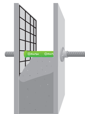
PASO 4: Adaptable a los diferentes grosores de muro
