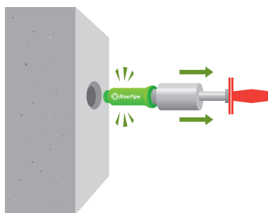
PASO 6: Extrae el RivePipe de los dos lados del muro
